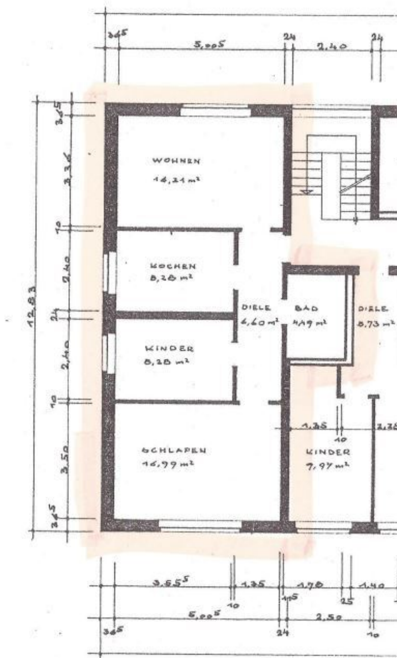
6403_Waldstr. 22_Grundriss
