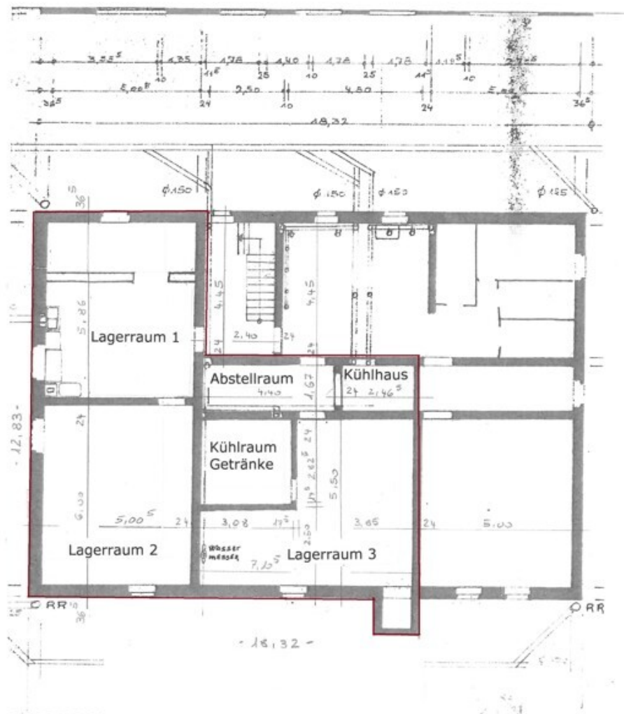
KELLERGESCHOSS
